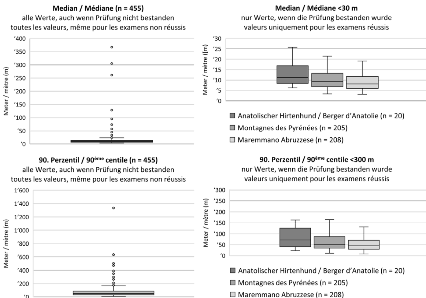
Illustration 1: Boîte à moustaches de la médiane des distances chien-moutons et 90 ème centile chien-moutons pour tous les chiens testés
